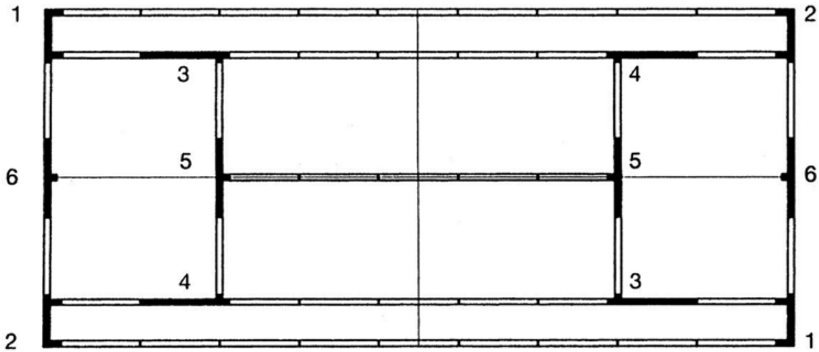
Verlegeplan ASS Tigerband
